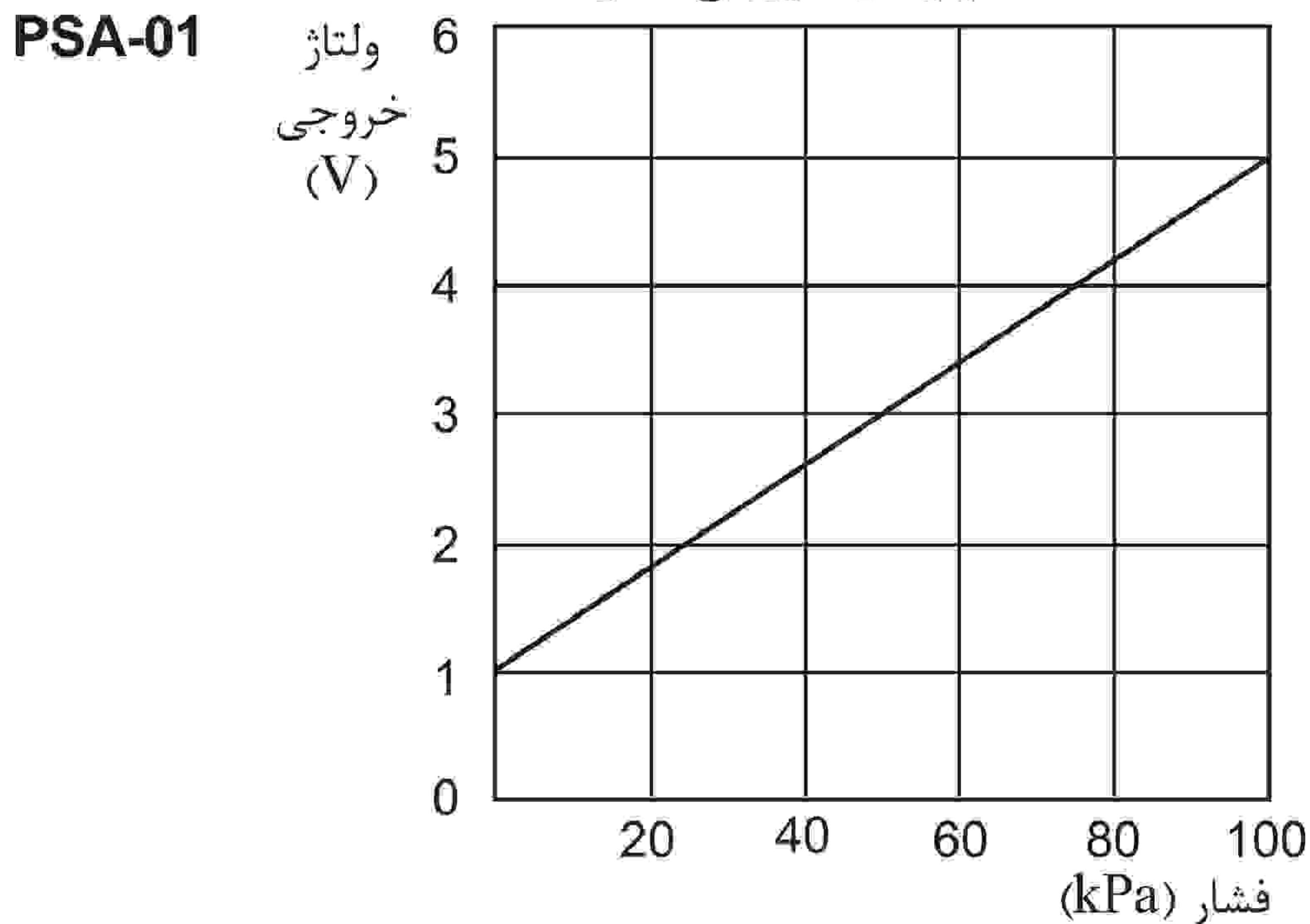
* مشخصه فشار ولتاژ خروجی آنالوگ
