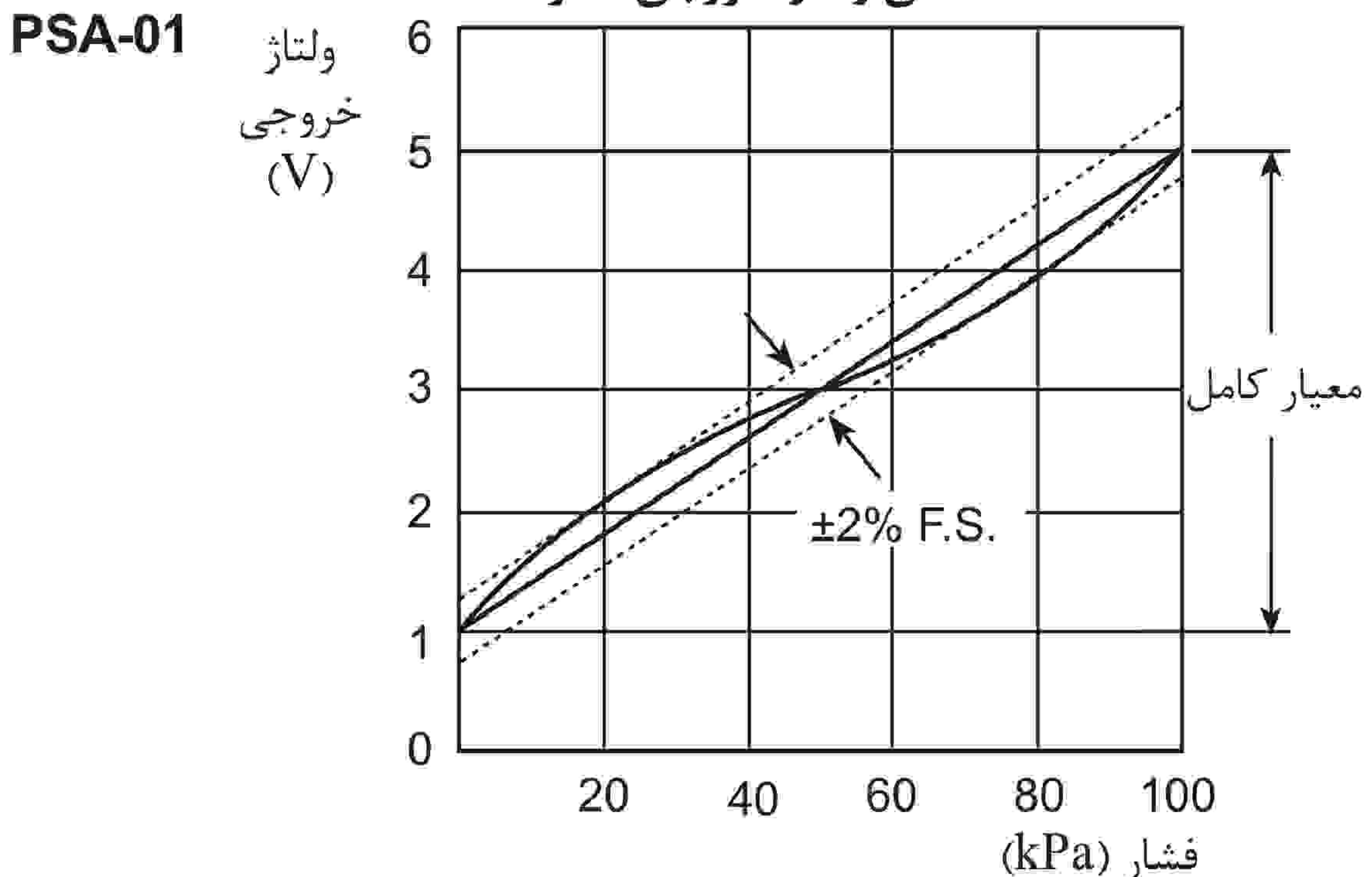
* مشخصه خطی ولتاژ خروجی آنالوگ
